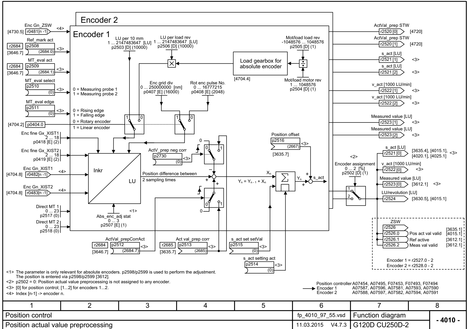
Fig. 3-100 4010 – Position actual value preprocessing
