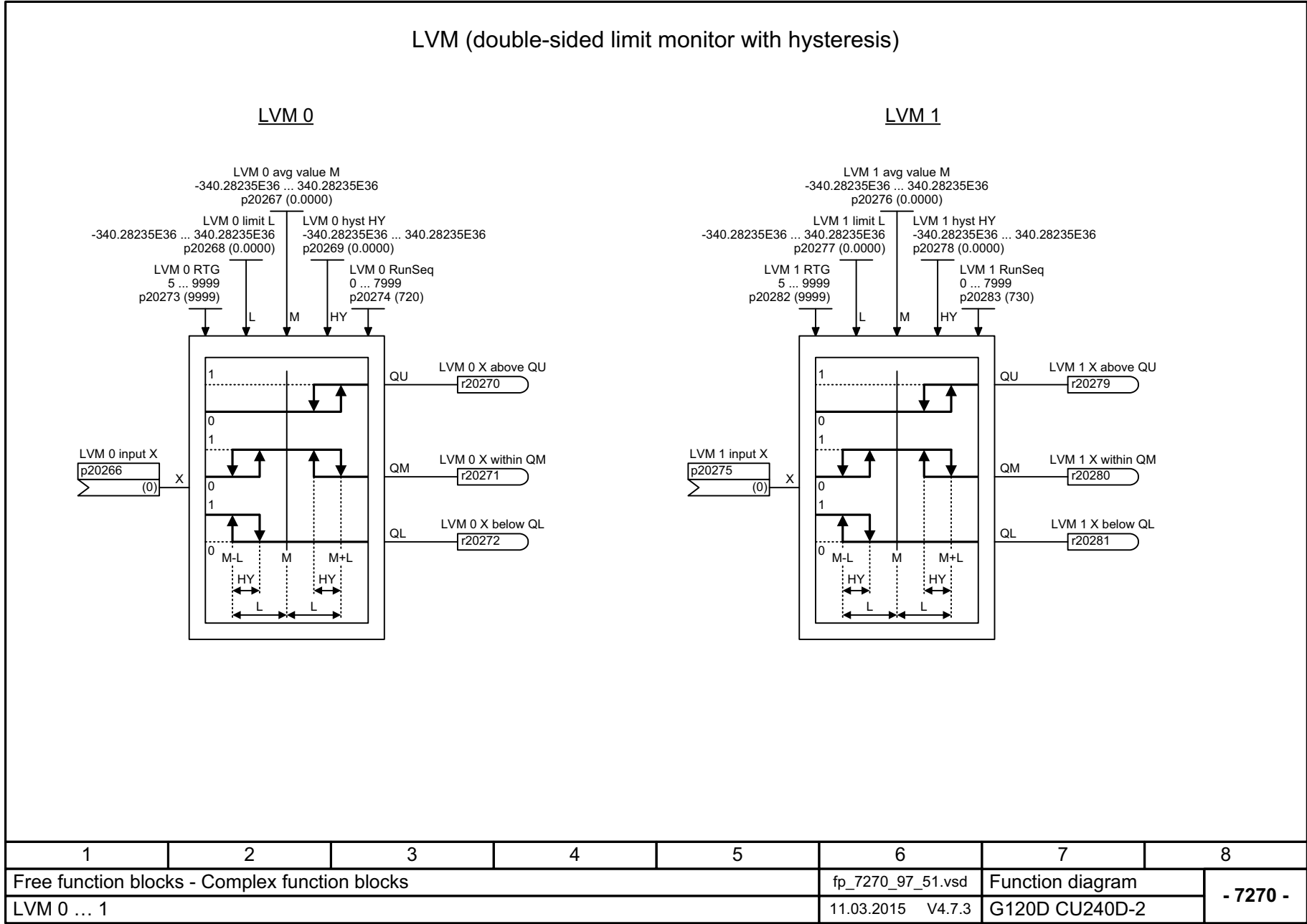
Fig. 3-154 7270 – LVM 0 ... 1
