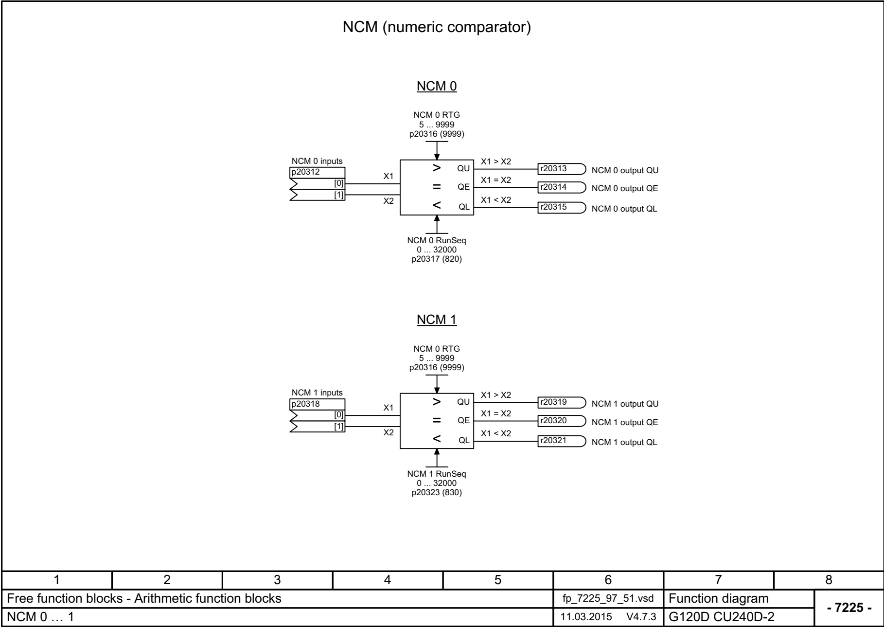
Fig. 3-143 7225 – NCM 0 ... 1
