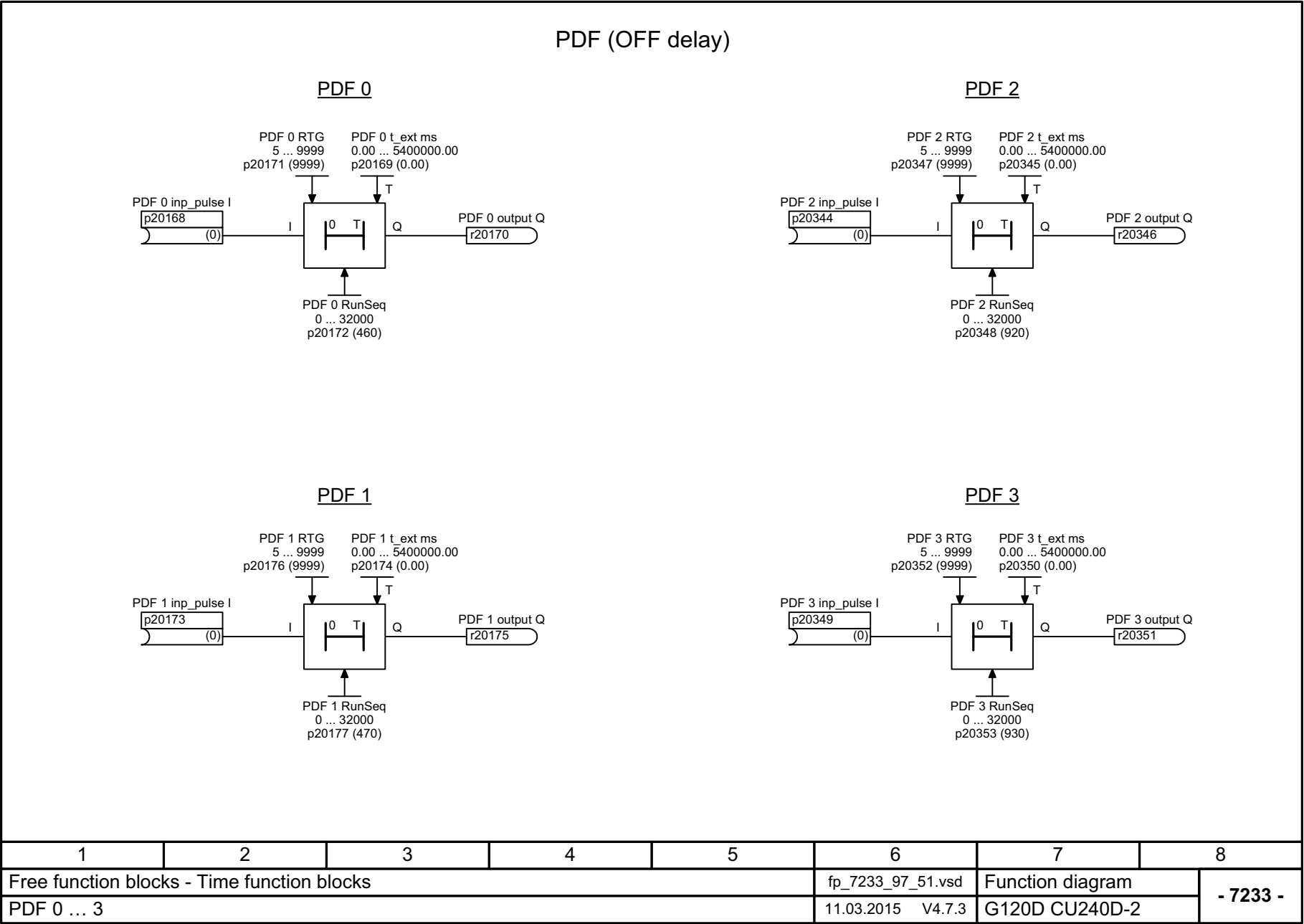
Fig. 3-147 7233 – PDF 0 ... 3
