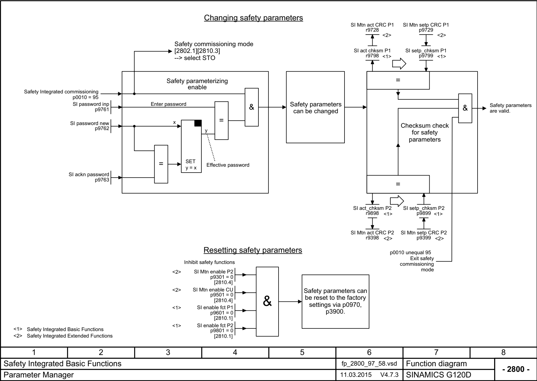
Fig. 3-57 2800 – Parameter manager
