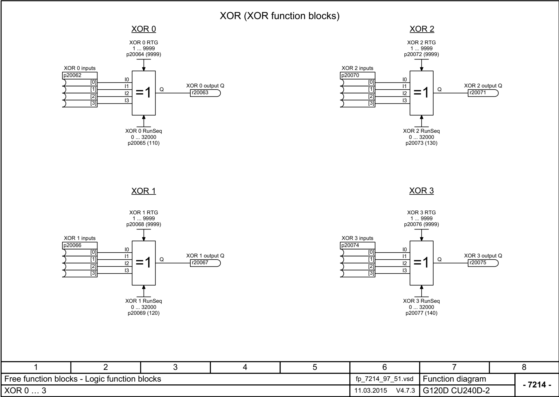
Fig. 3-138 7214 – XOR 0 ... 3
