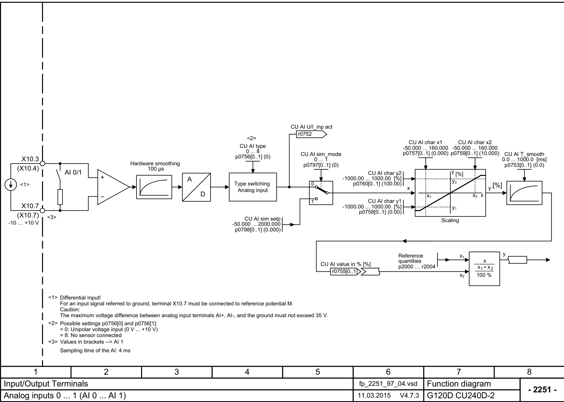
Fig. 3-8 2251 – Analog inputs (AI 0 ... AI 1)
