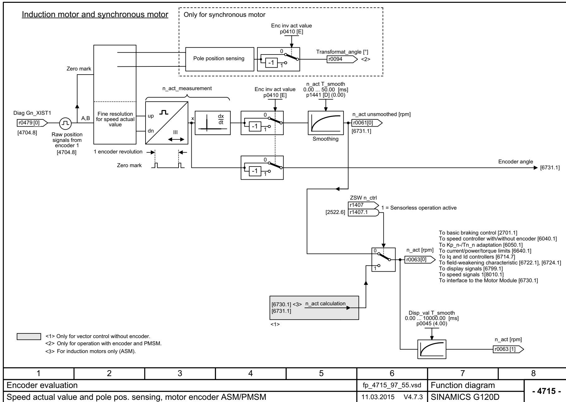
Fig. 3-105 4715 – Speed actual value and pole pos. sensing, motor encoder ASM/SM (encoder 1)
