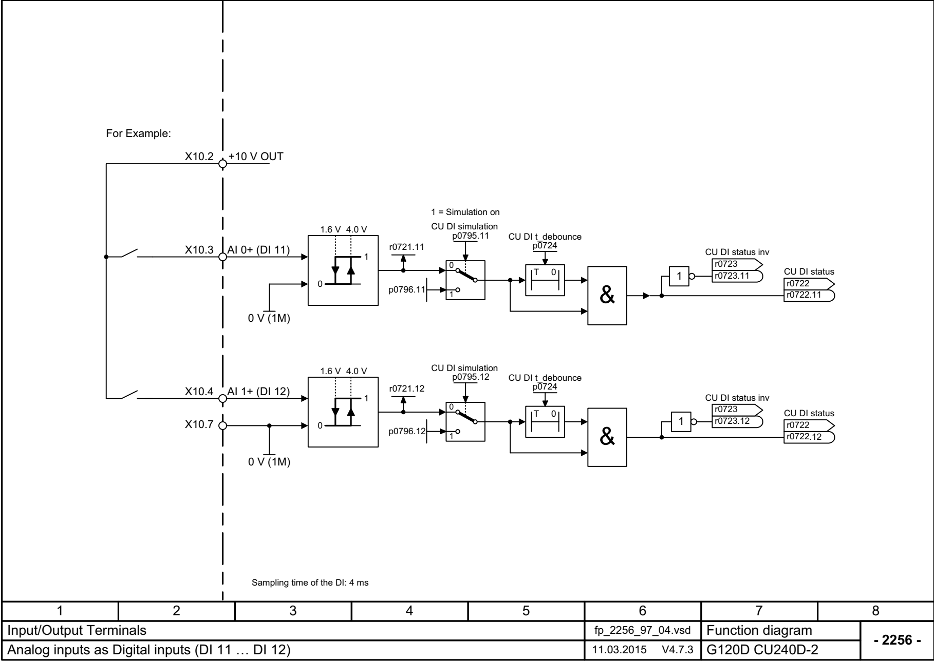
Fig. 3-9 2256 – Analog inputs as digital inputs (DI 11 ... DI 12)
