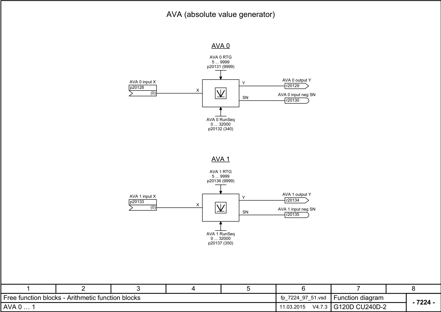
Fig. 3-142 7224 – AVA 0 ... 1
