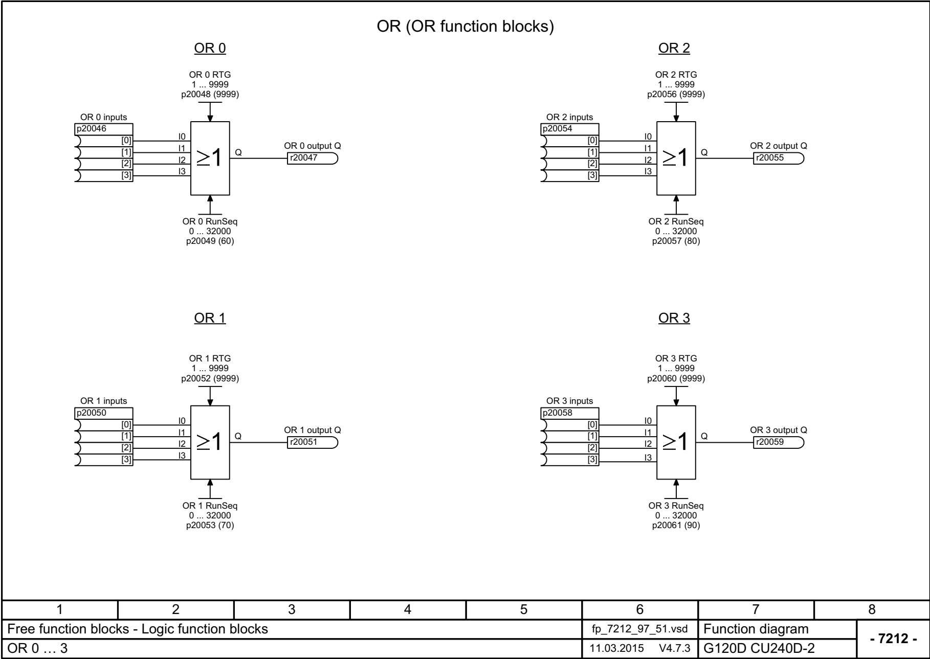
Fig. 3-137 7212 – OR 0 ... 3
