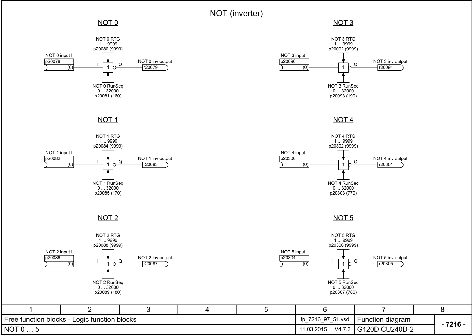
Fig. 3-139 7216 – NOT 0 ... 5
