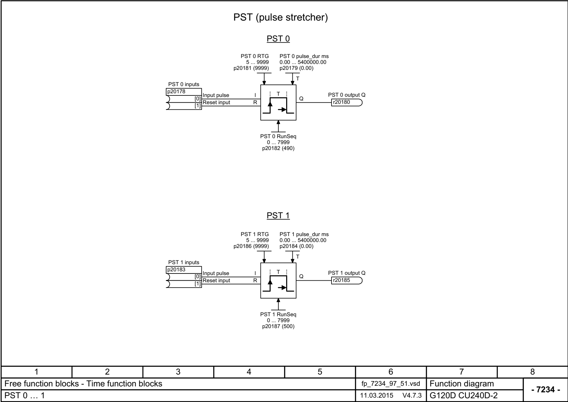
Fig. 3-148 7234 – PST 0 ... 1
