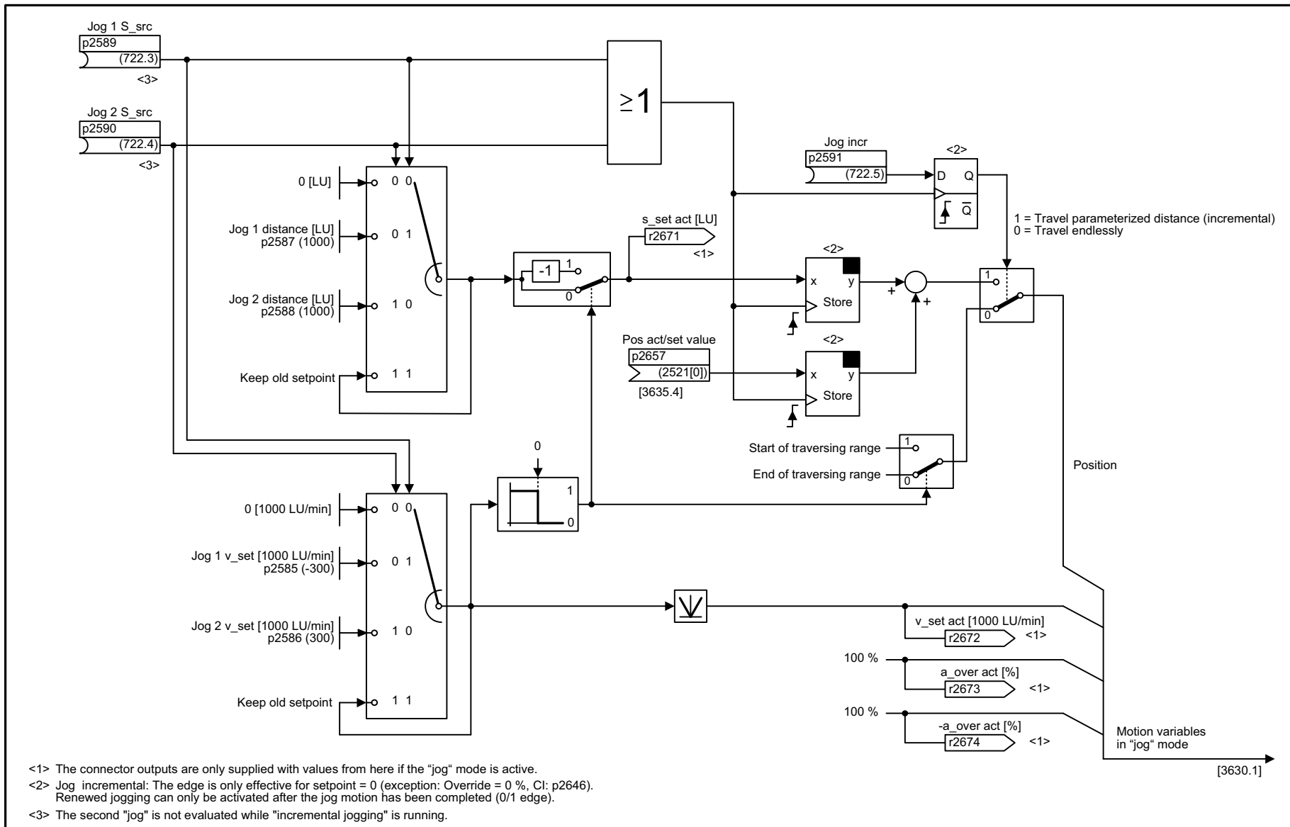
Fig. 3-85 3610 – Jog mode
