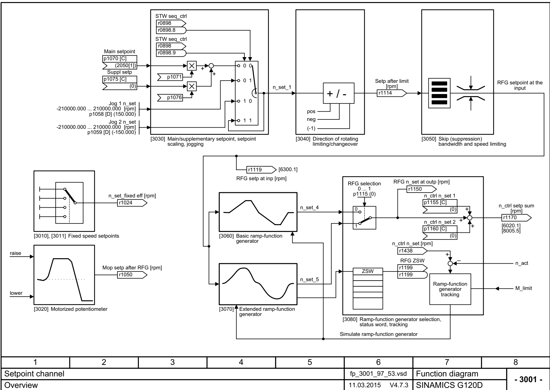
Fig. 3-75 3001 – Overview
