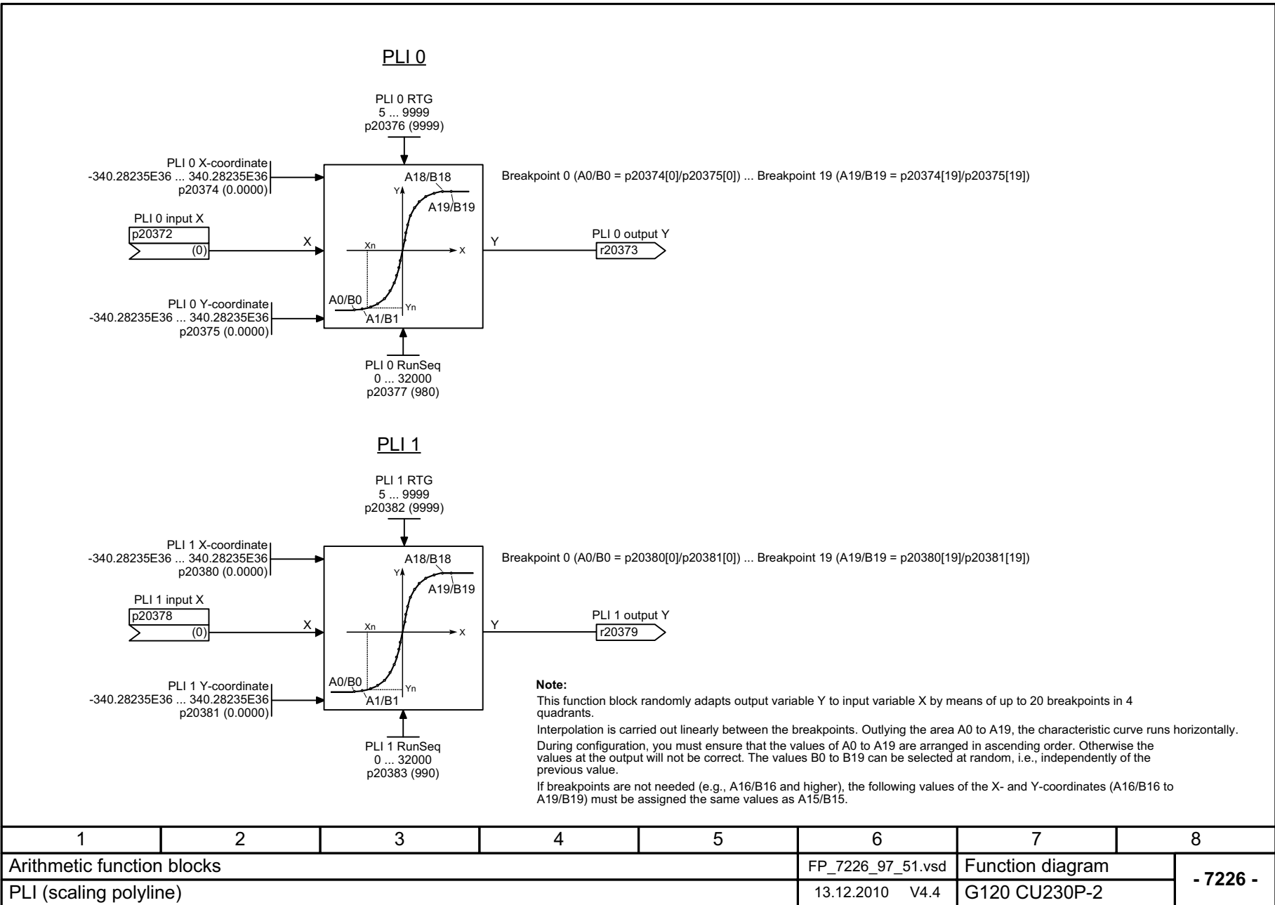
Fig. 2-101 7226 – PLI (scaling polyline)
