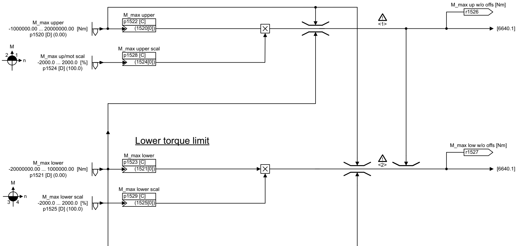
Fig. 2-81 6630 – Upper/lower torque limit
