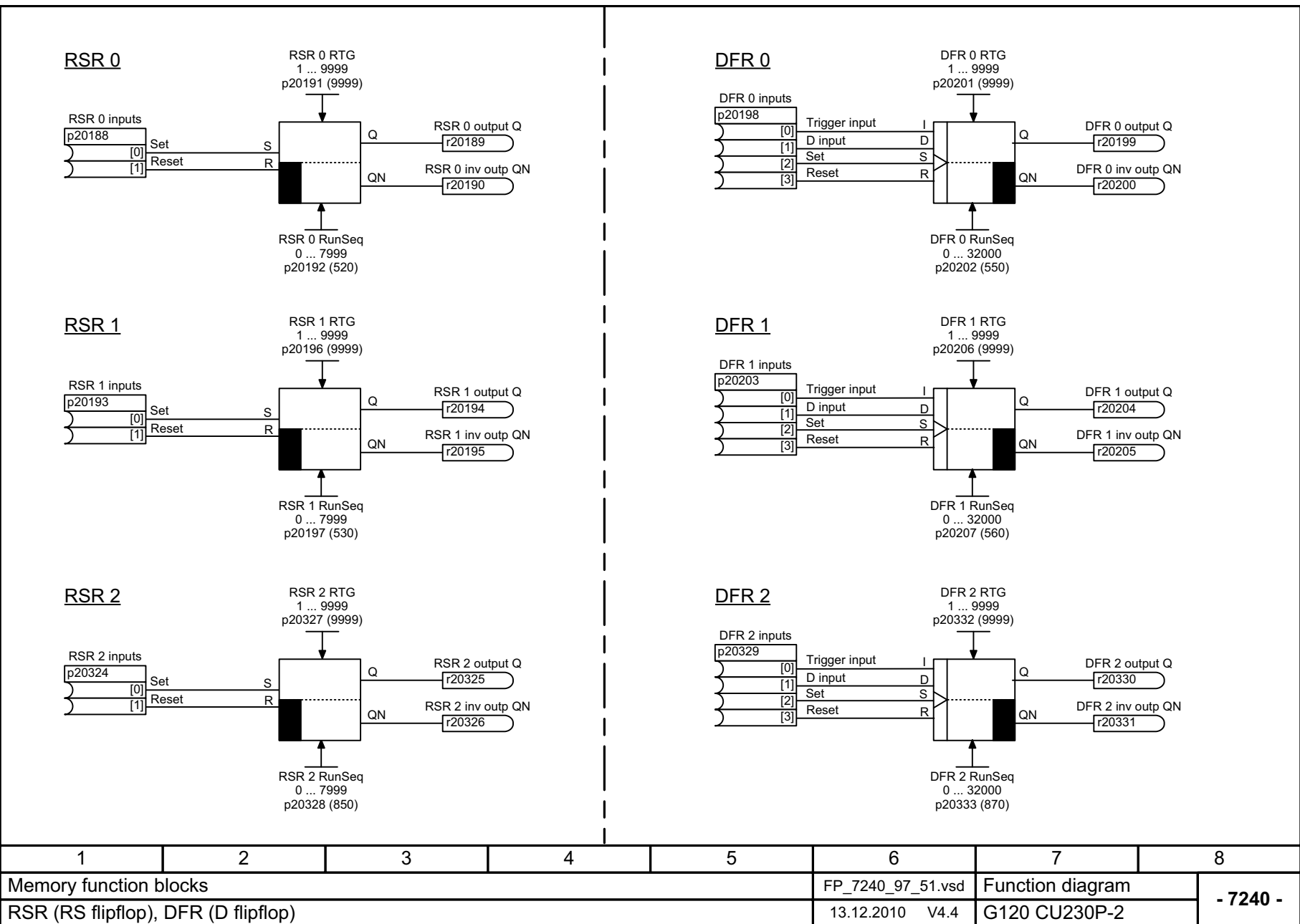
Fig. 2-106 7240 – RSR (RS flipflop), DFR (D flipflop)
