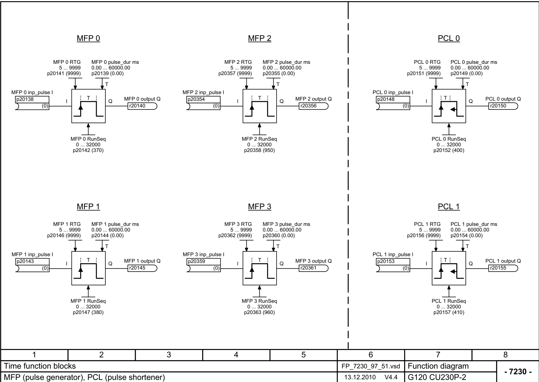
Fig. 2-102 7230 – MFP (pulse generator), PCL (pulse shortener)
