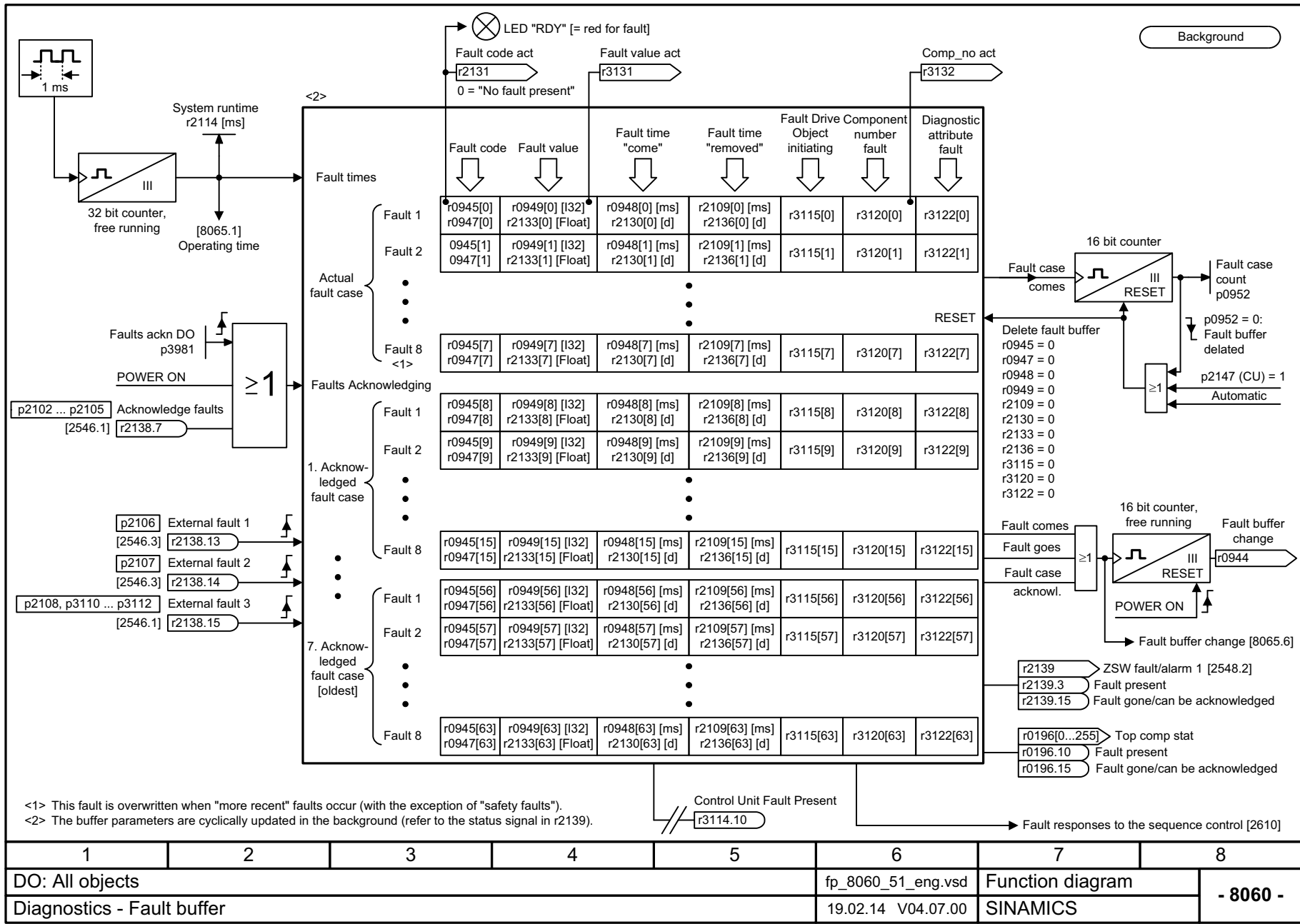
Fig. 3-162 8060 – Fault buffer
