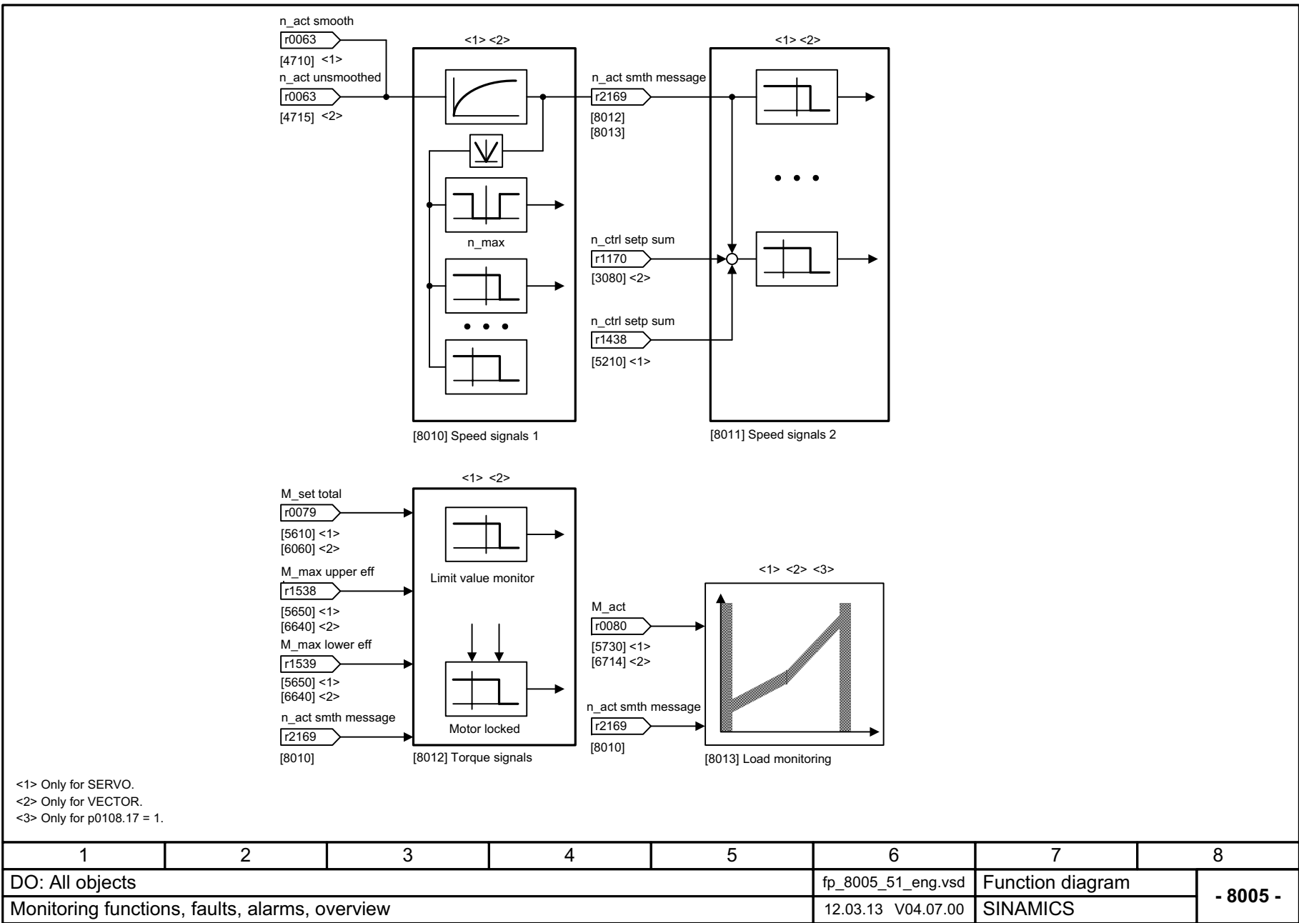
Fig. 3-153 8005 – Overview
