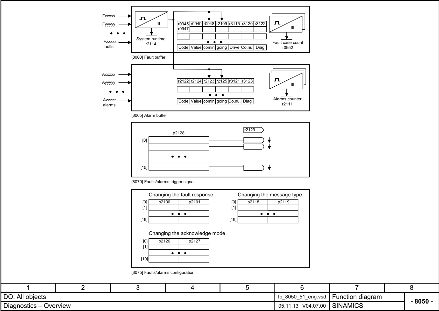
Fig. 3-161 8050 – Overview
