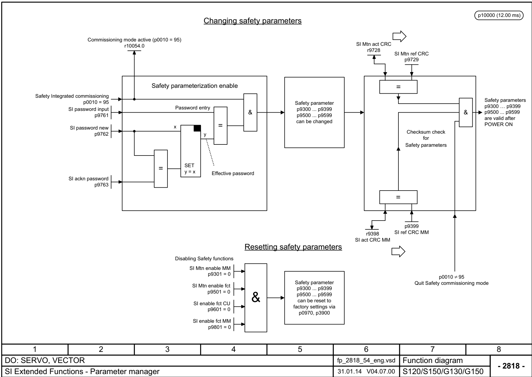
Fig. 3-82 2818 – Parameter manager
