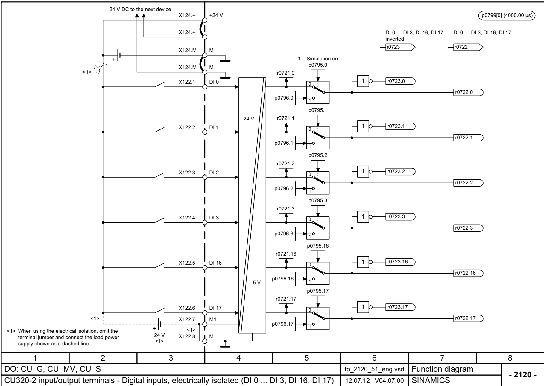
Fig. 3-6 2120 – Digital inputs, electrically isolated (DI 0 ... DI 3, DI 16, DI 17)
