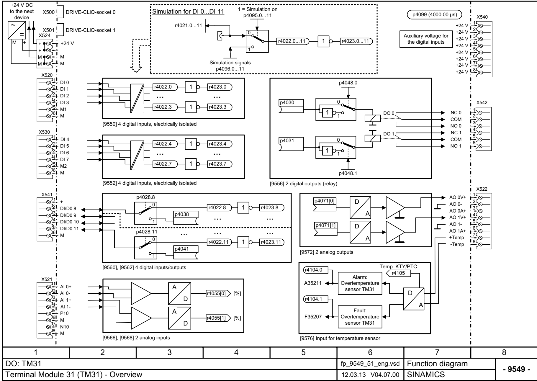
Fig. 3-190 9549 – Overview
