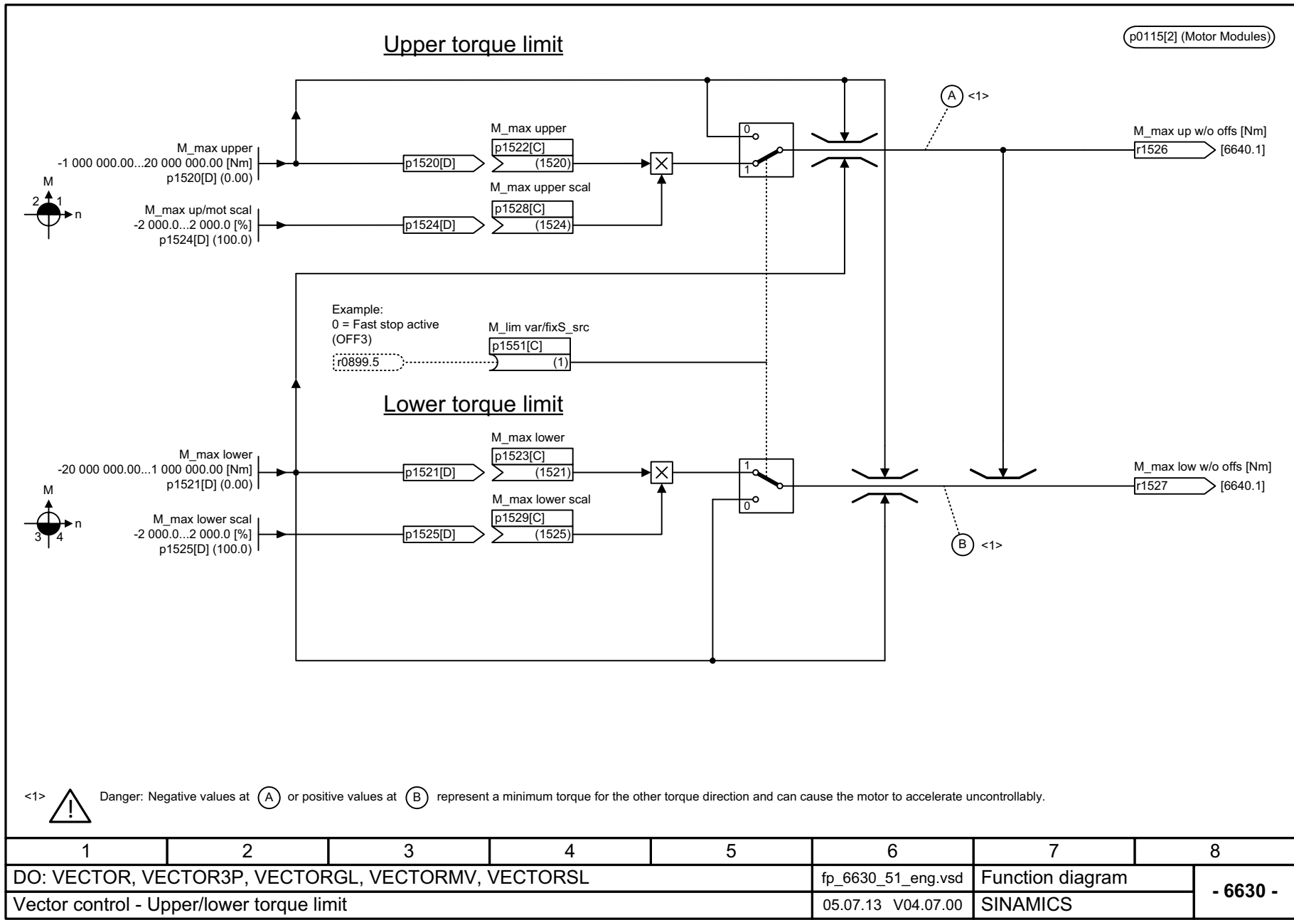
Fig. 3-130 6630 – Upper/lower torque limit
